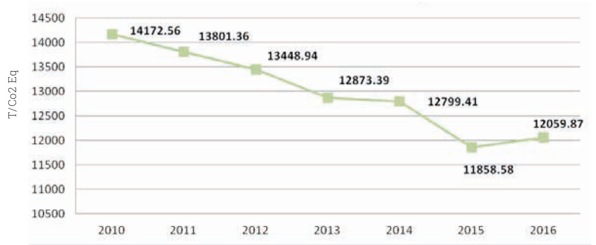
Yıllara Göre Kurumsal Sera Gazı Değerleri
